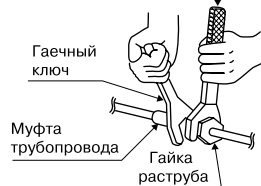
Гаечный ключ с ограничением по крутящему моменту
